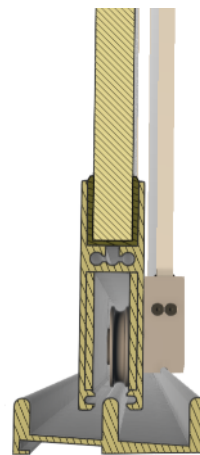
Boční řez 3-drážkovou kolejnicí včetně pojezdového profilu a zasklení s gumou
